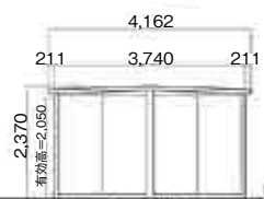
【立面図】
